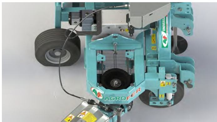
Tárcsák ékszíjas meghajtása
