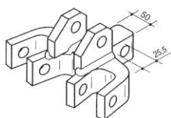
Csatlakozó elem 3.pont függesztéshez és feszítő-csavarokhoz
