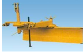
A 45.2 és 55.2 szériáknál a lap 360°-ban, a függesztés 180°-ban állítható
