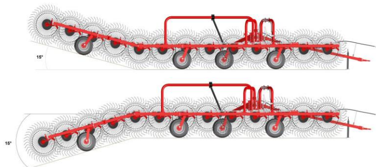
A csuklós váz \pm 15^\circ -ban mozoghat
